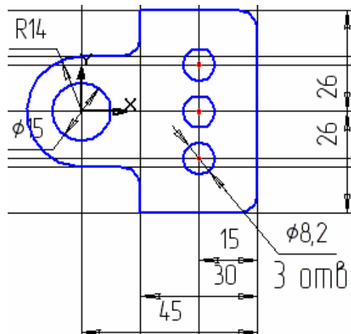
Рис. 3.9. Построение дуги
