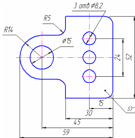
Рис. 3.1. Чертеж подвески
